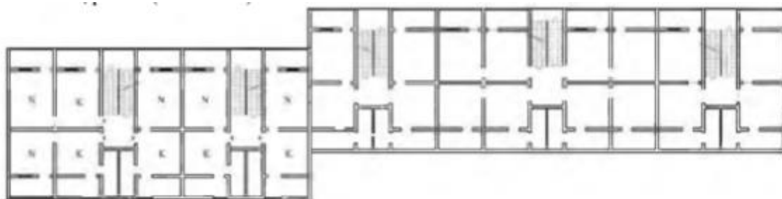
Hình 2.21. Mặt bằng dãy nhà Khu tập thể Thanh Xuân kiểu đơn nguyên
