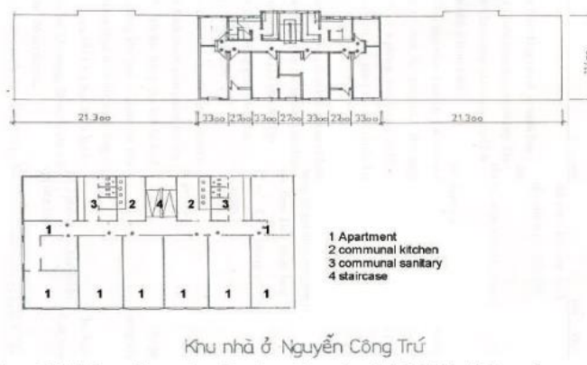
Hình 2.11. Thiết kế khu nhà ở Nguyễn Công Trứ
