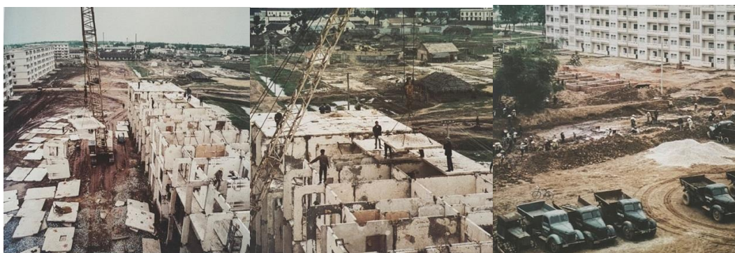
Hình 4.7. Quá trình lắp ghép Khu tập thể Trung Tự năm 1975
