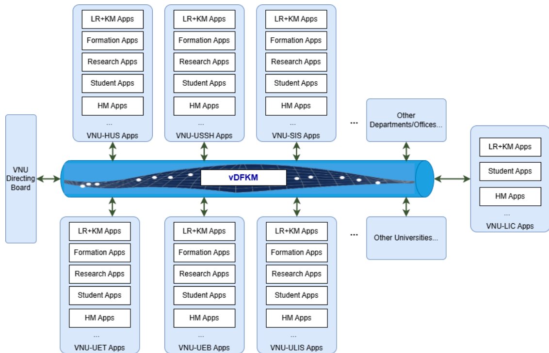
Hình 4.2: Mô hình triển khai vDFKM trong toàn hệ thống ĐHQGHN
