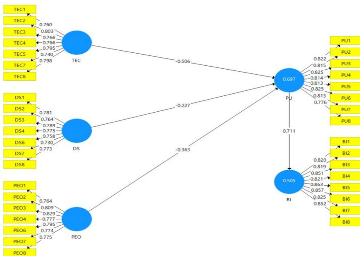
Hình 3.9: Mô hình cấu trúc sau khi tinh chỉnh thang đo ( R^2_{PU} = 0.697 , R^2_{BI} = 0.505 ).
