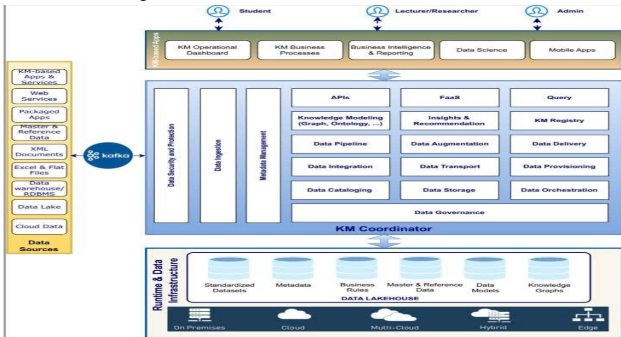
Hình 4.1: Khung quản lý tri thức vDFKM
