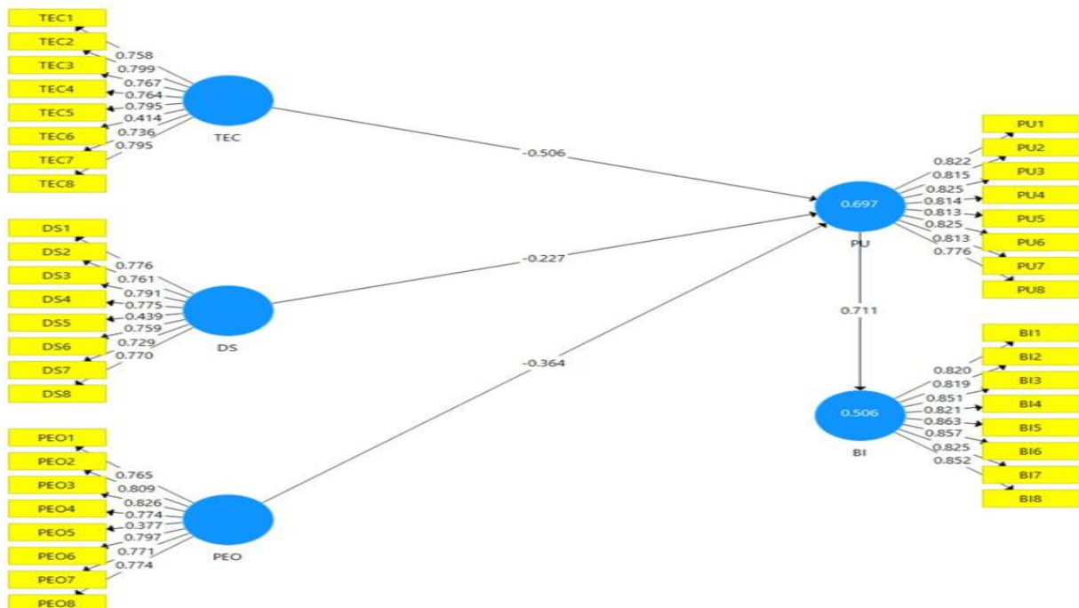
Hình 3.8: Mô hình cấu trúc trước khi tinh chỉnh thang đo ( R^2_{PU} = 0.697 , R^2_{BI} = 0.506 ).
