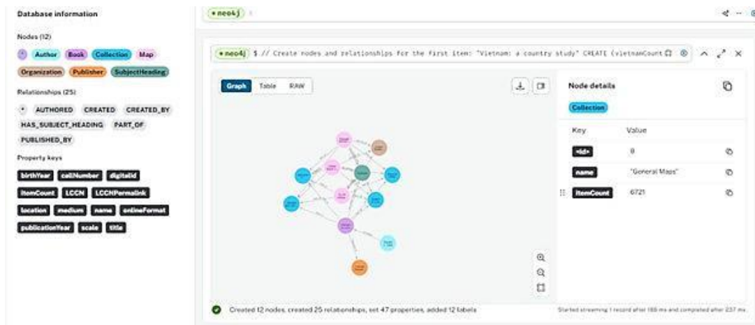
Hình 4.4: Truy vấn Cypher và Đồ thị trong ngữ cảnh: Việt Nam - một quốc gia
